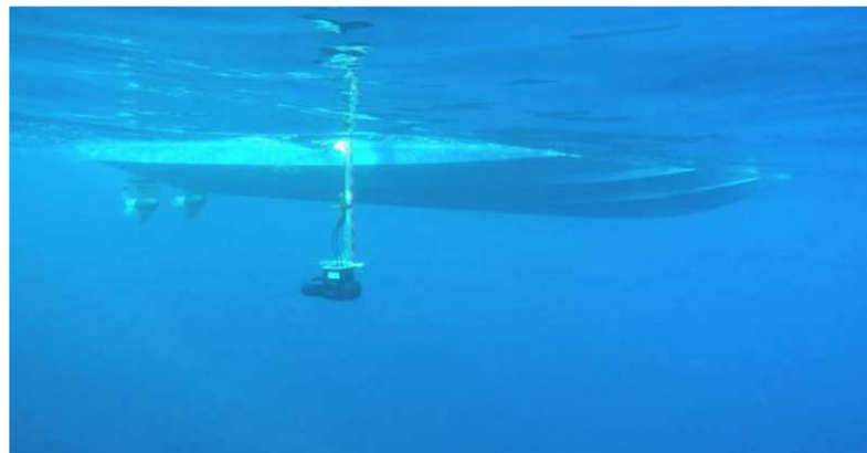
SMF Norbit iWBMSH intégré au système déployable d'hydrographie
