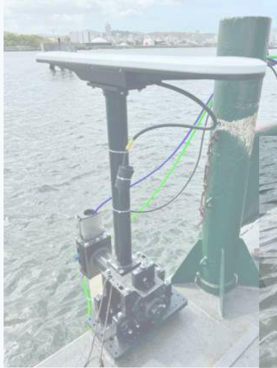
Kongsberg EM 2040P
